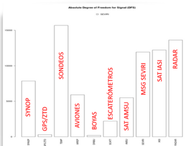
Fig. 5.10 – Impacto de las distintas observaciones en el análisis operativo de HARMONIE-AROME medido con el indicador Absolute Degree of Signal (DFS).
