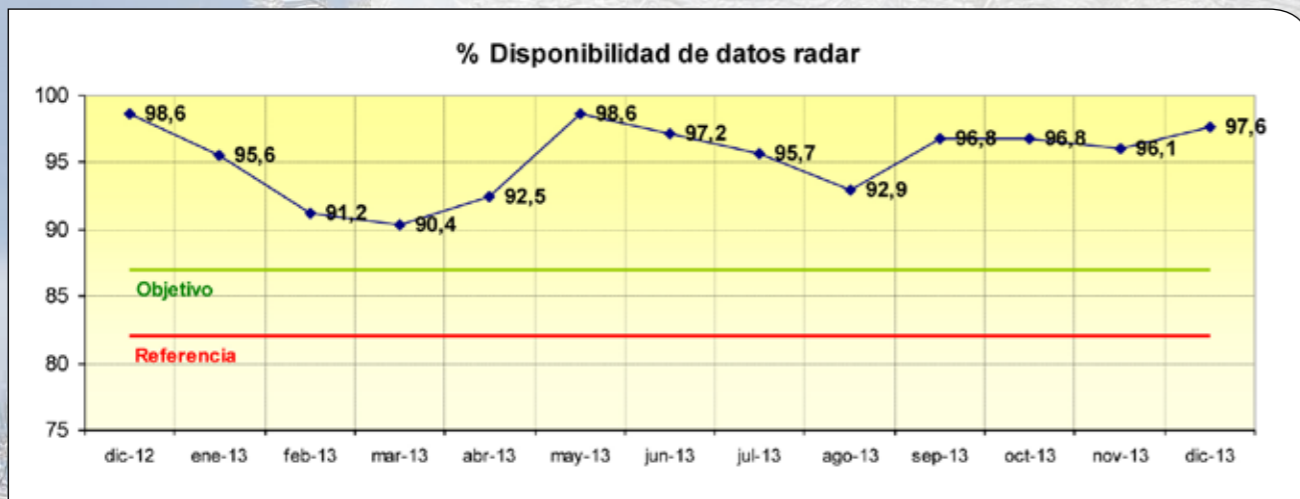
Disponibilidad de datos de la red de radares de AEMET a lo largo de 2013
